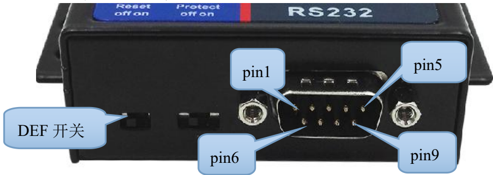
图 5 RS232 接口和拨码
