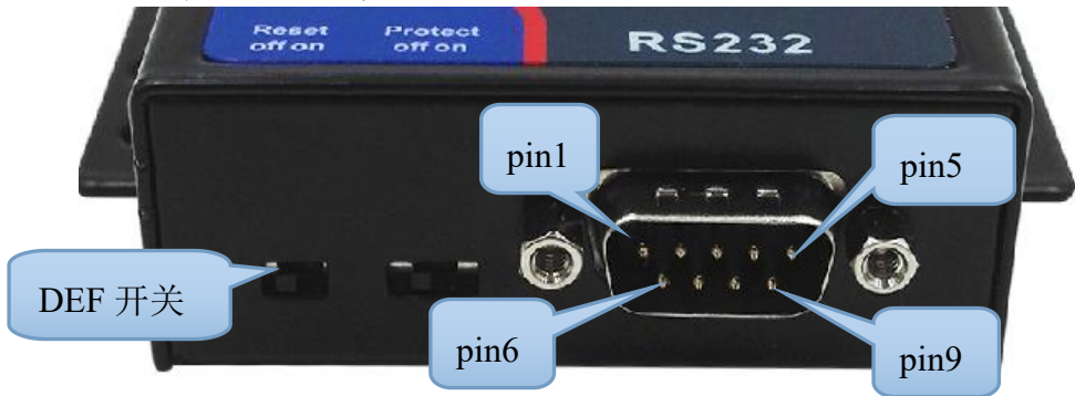
图 5 RS232 接口和拨码
