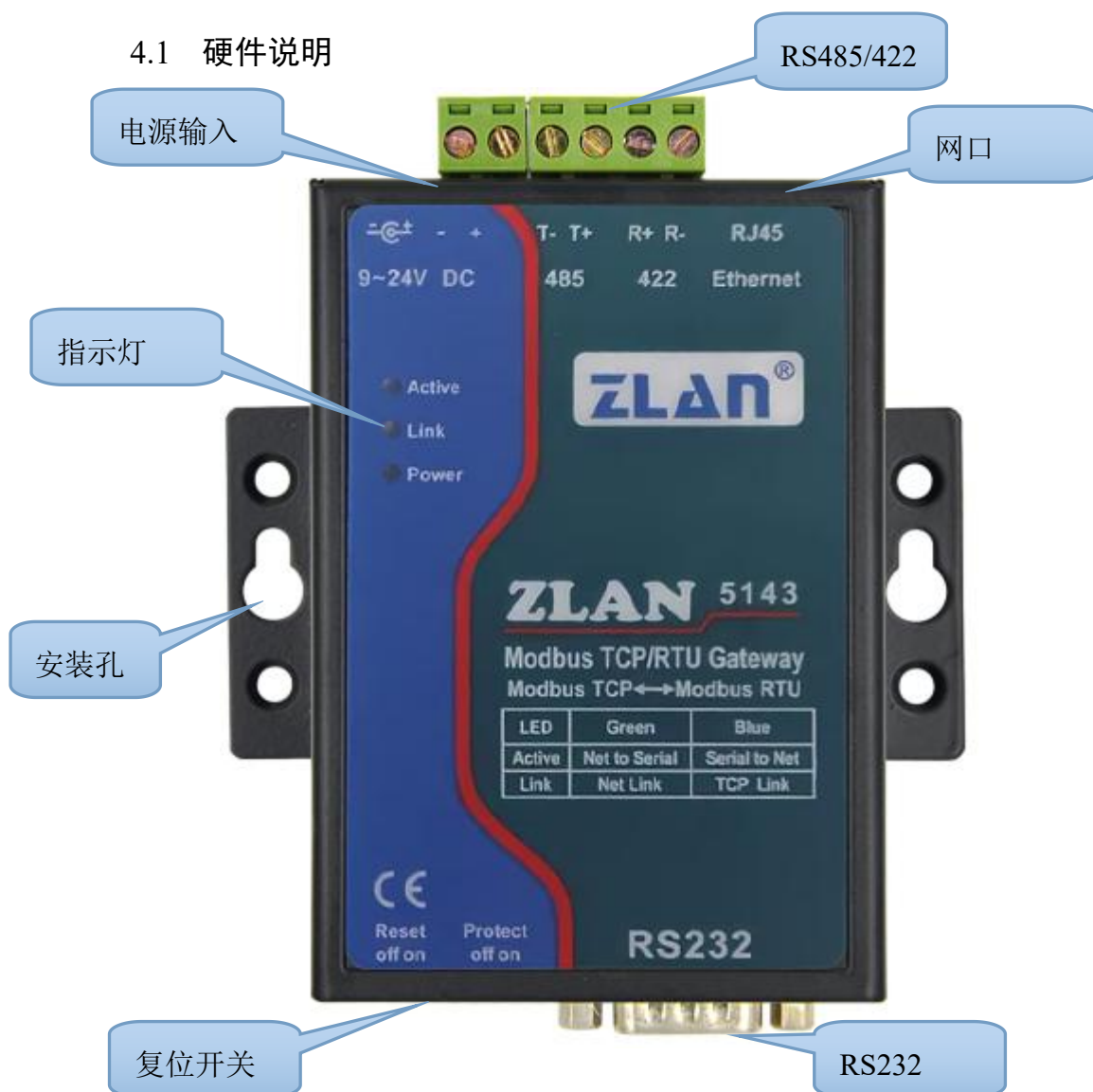
图 3 正视图
