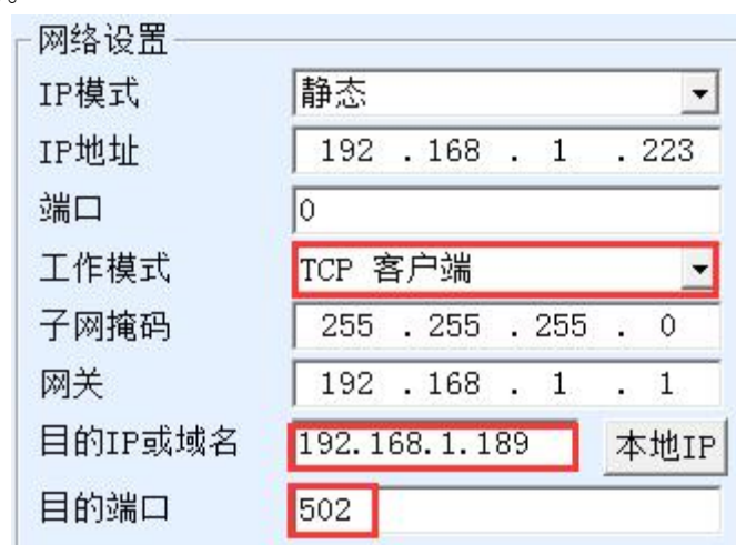
图 24 Modbus TCP 做客户端
