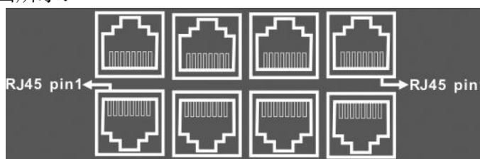
图 6 网线线序
