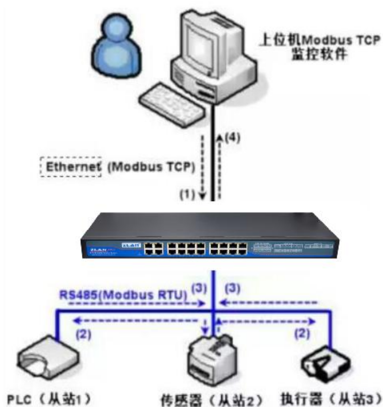
图 40 存储型 Modbus 网关工作方式
