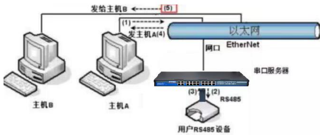
图 42 多主机功能演示
