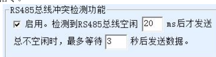
图 44 RS485 防冲突空闲时间
