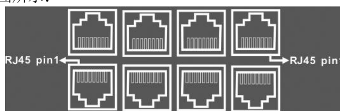
图 6 网线线序
