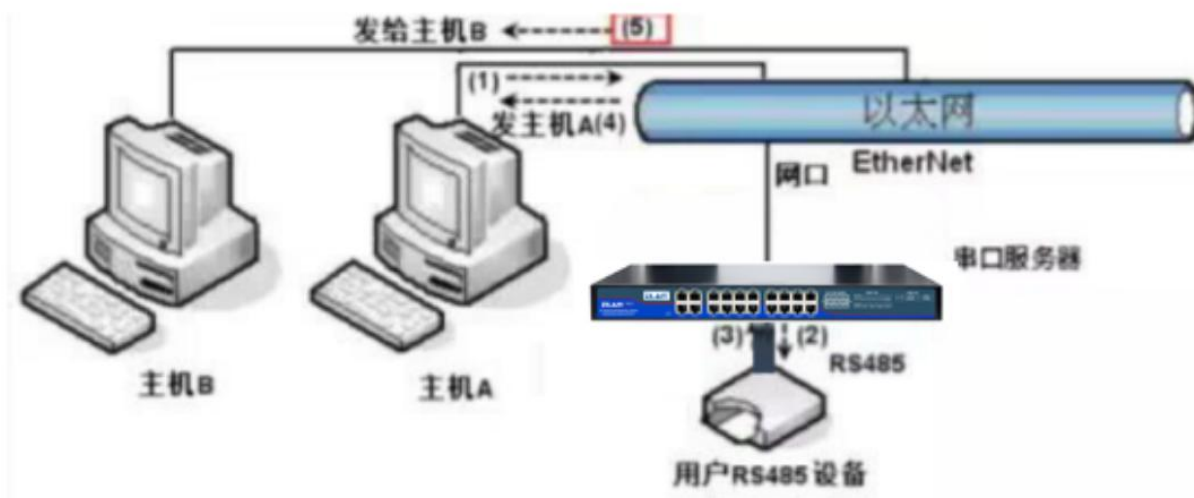
图 42 多主机功能演示
