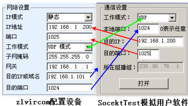
图 33 UDP 模式参数配置
