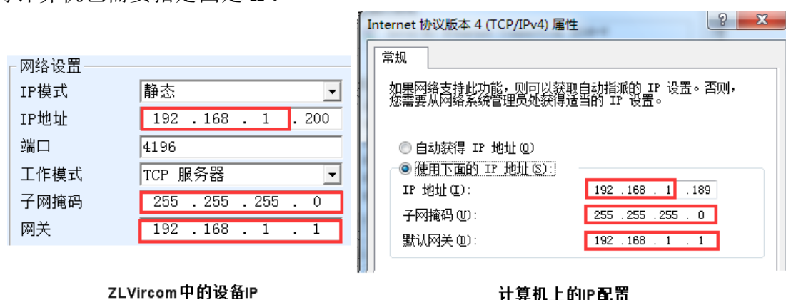
图 37 配置在同一个网段
