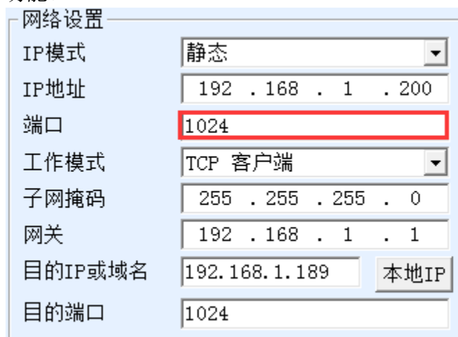
图 32 既做客户端也做服务器
