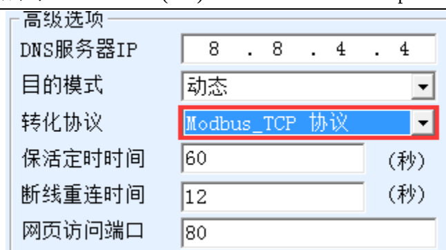
图 24 启用 Modbus TCP 功能
