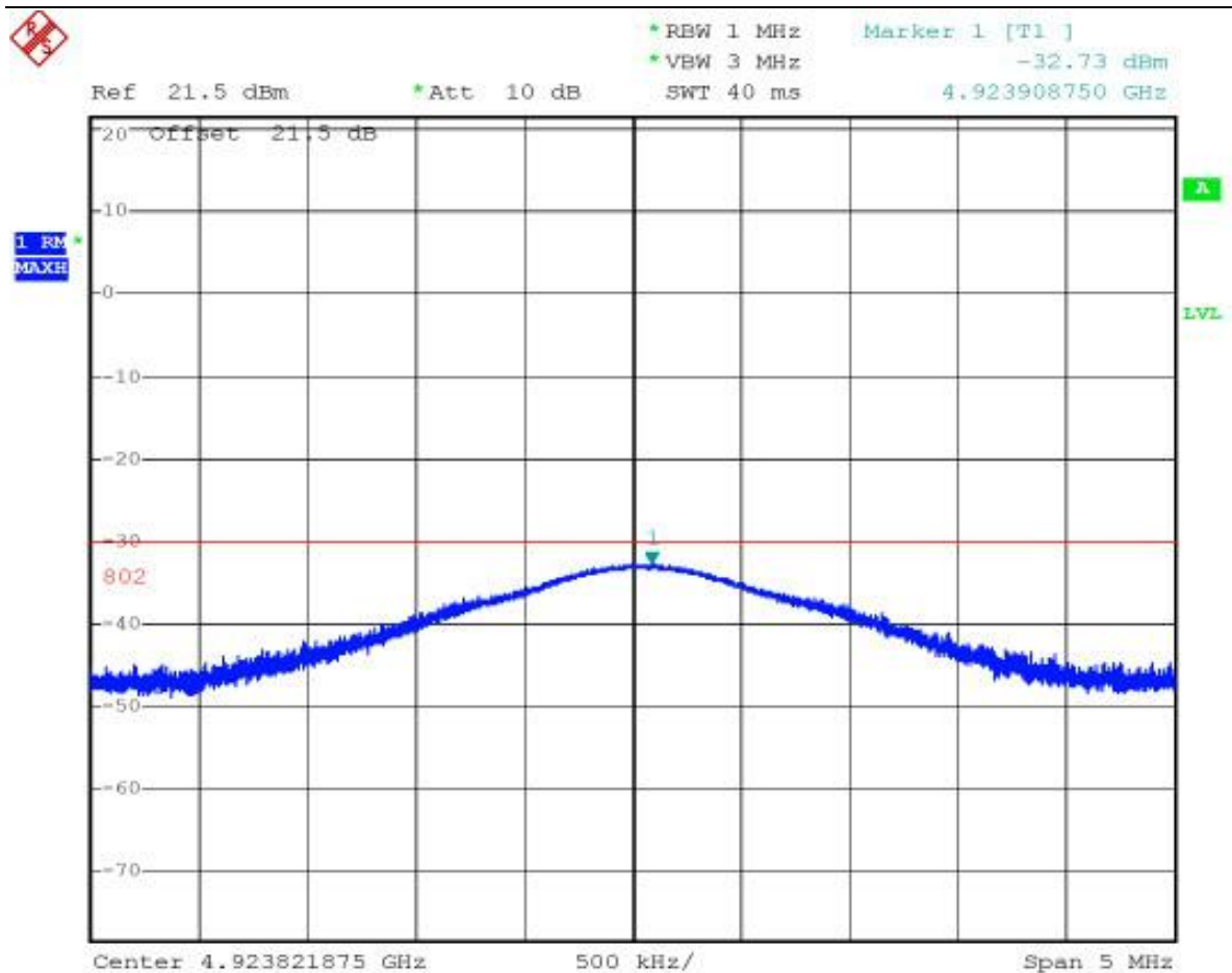
图 13 7004 杂散测试曲线
