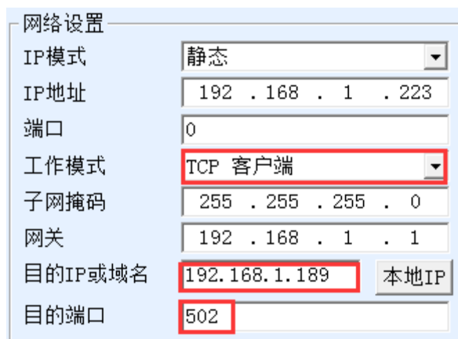
图 25 Modbus TCP 做客户端。
