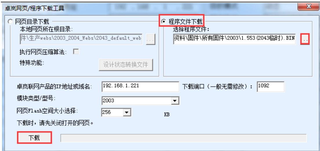
图 58 ZLSN2003 固件升级方法
