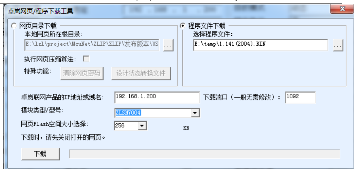
图 59 ZLSN2003 web 升级方法
