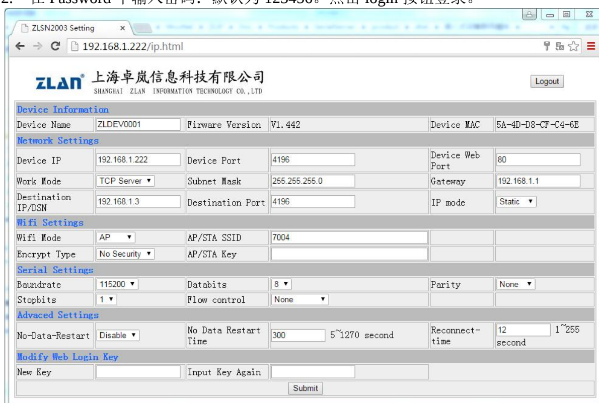
图 27 Web 配置界面
