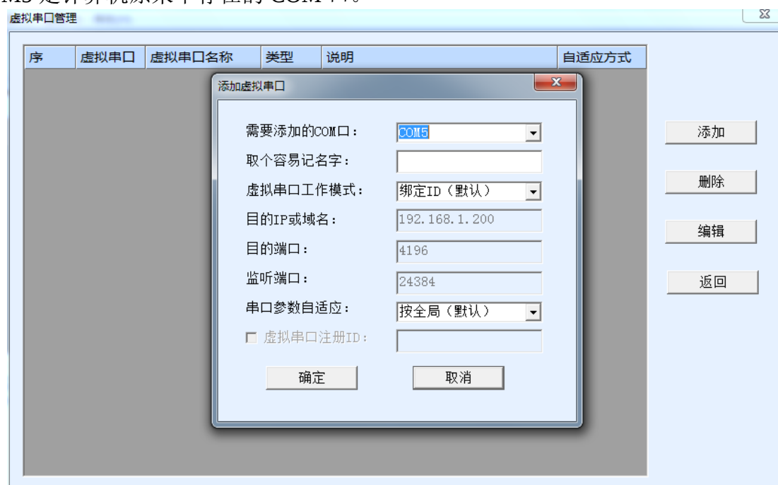
图 21 添加虚拟串口
