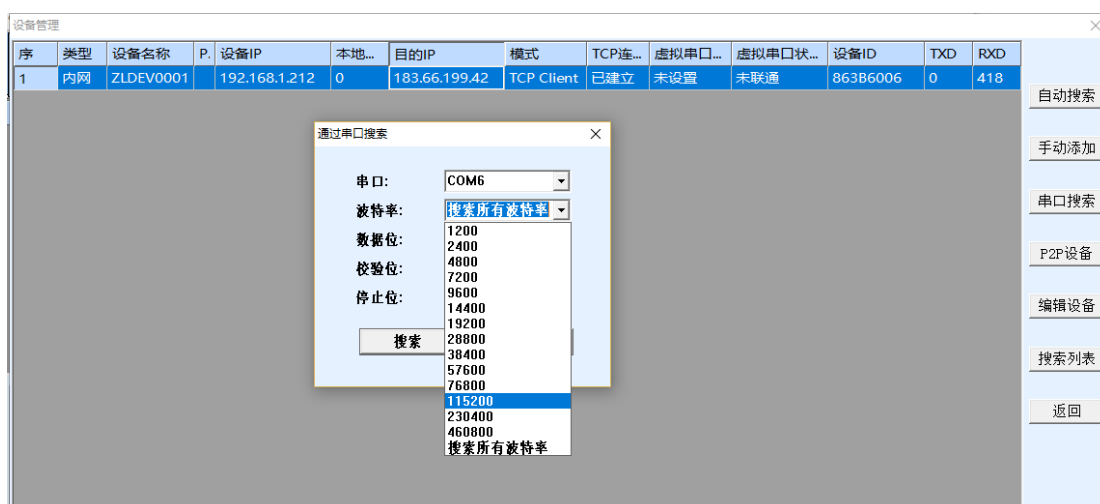
图 7 串口配置工具
