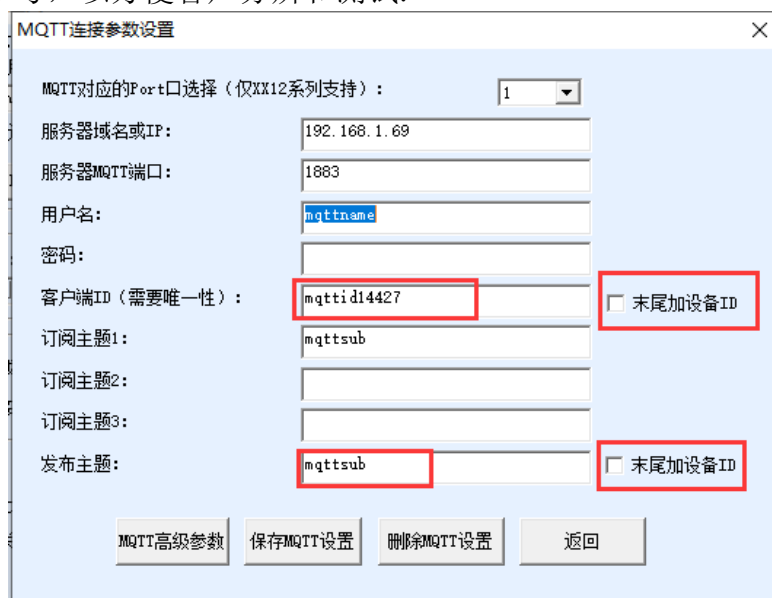
图 42 mqtt 自动增加设备 ID
